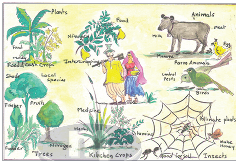
Figure 11.1 Biodiversity
